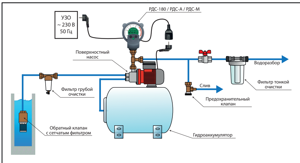
Пример 1. Подключение РДС к поверхностному насосу или насосной станции.
