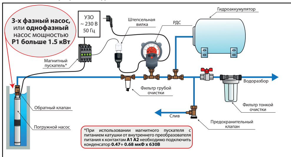
Пример 4. Подключение РДС для управления однофазным насосом мощностью P1 более 1.5 кВт, или трехфазным погружным насосом.
