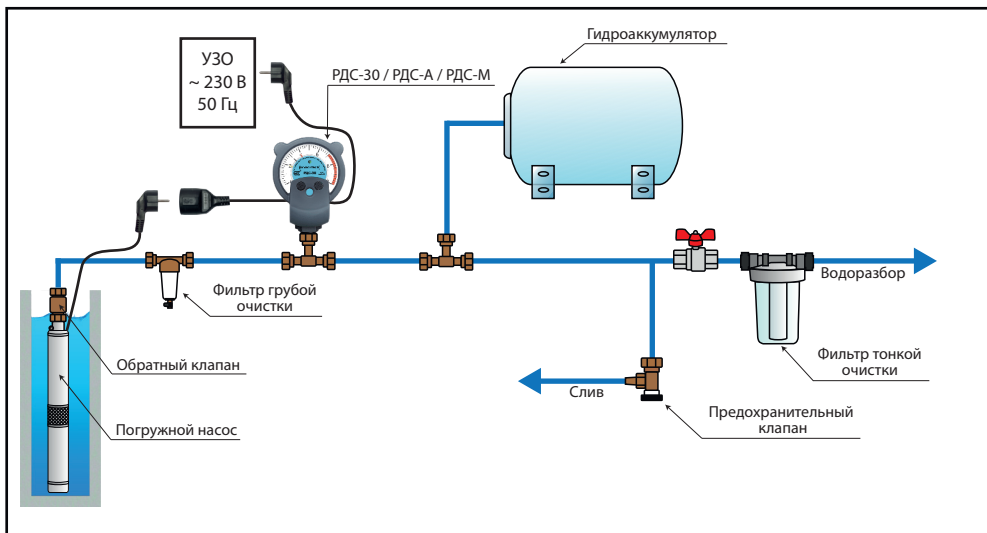
Пример 2. Подключение РДС к погружному насосу.
