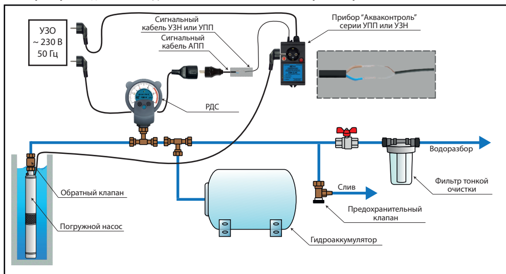
Пример 3. Подключение РДС к УПП или УЗН "Extra Акваконтроль" через АПП.
